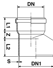
Excéntrico
