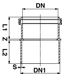
Concéntrico
