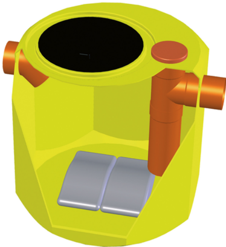
Arqueta con filtro oleoabsorbente
