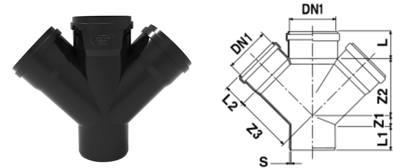
Derivación doble 45° macho-hembra
