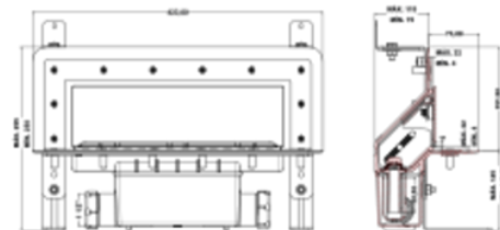
Embelledor acero inox y ABS
