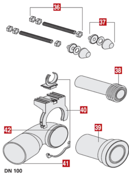
Junta curva evacuación 90°
