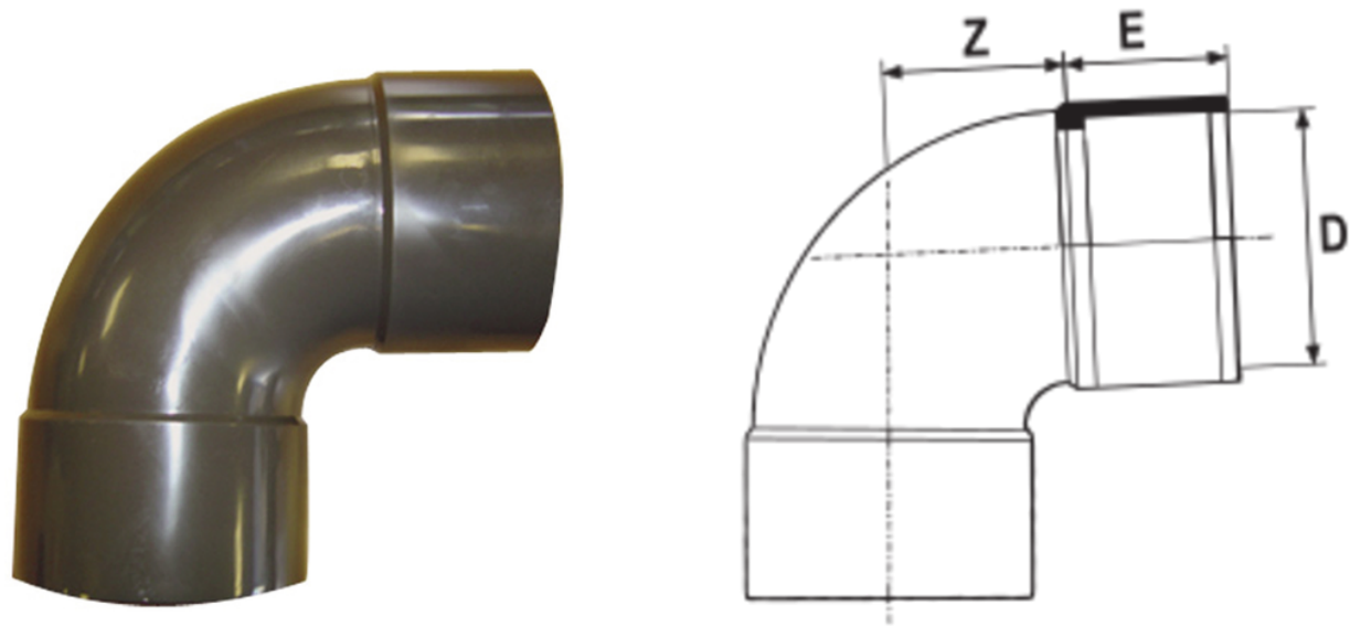
Codo 90° Hembra – Hembra HTA-E
