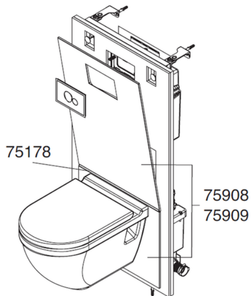
Placa frontal cristal
