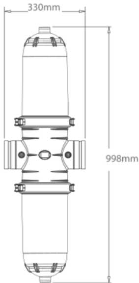
Filtro 100 micras hidrociclónico doble cuerpo compacto-ANILLAS
