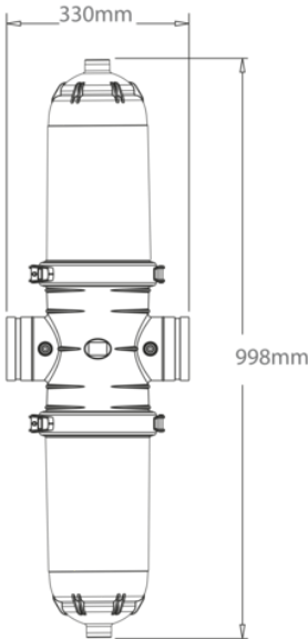
Filtro 50 micras hidrociclónico doble cuerpo compacto-ANILLAS
