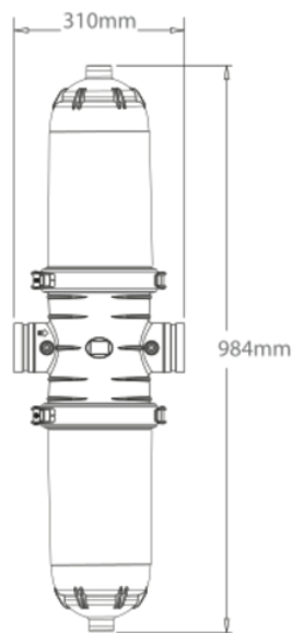
Filtro 100 micras hidrociclónico doble cuerpo compacto-ANILLAS
