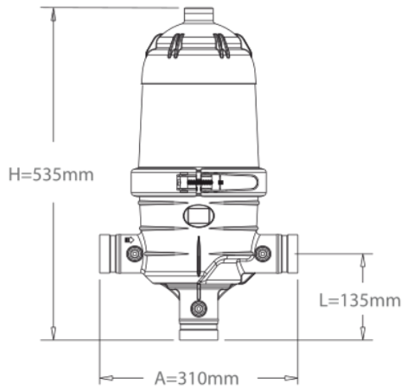
Filtro 50 micras hidrociclónico-ANILLAS
