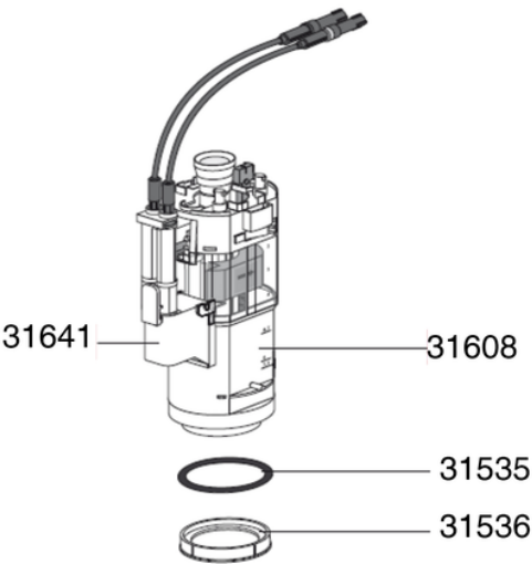
INEO – Junta mecanismo descarga
