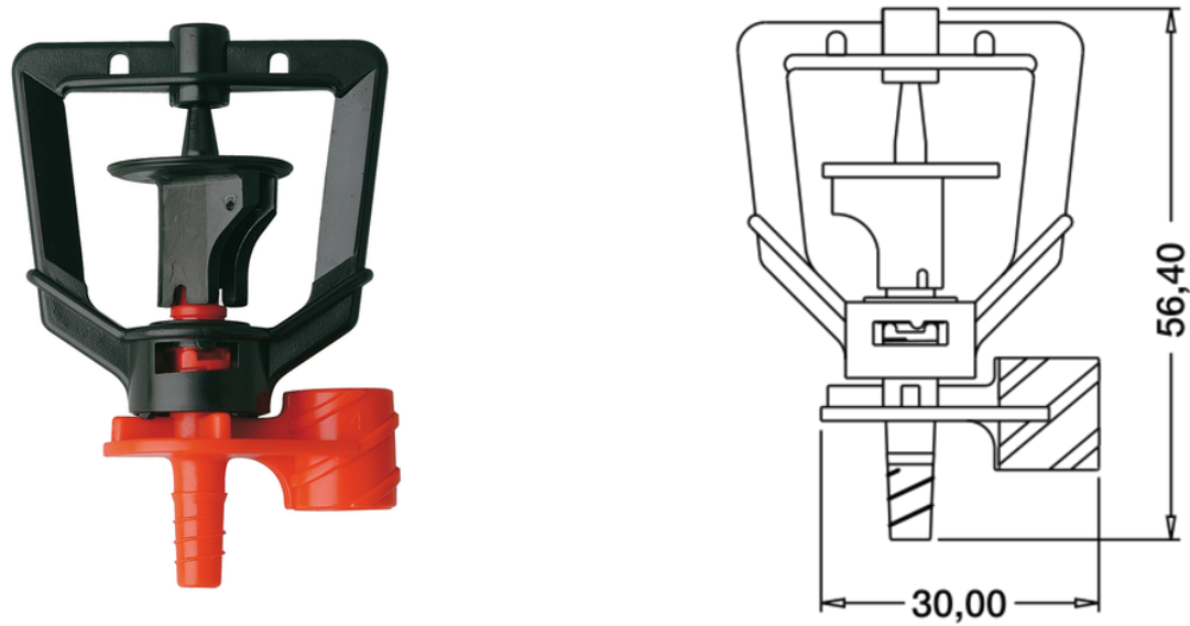
Microaspersor sin regulación de caudal
