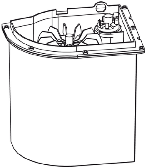
Conjunto casete estación bombeo - CICLON LS
