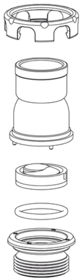
Conjunto válvula impulsión - CICLON
