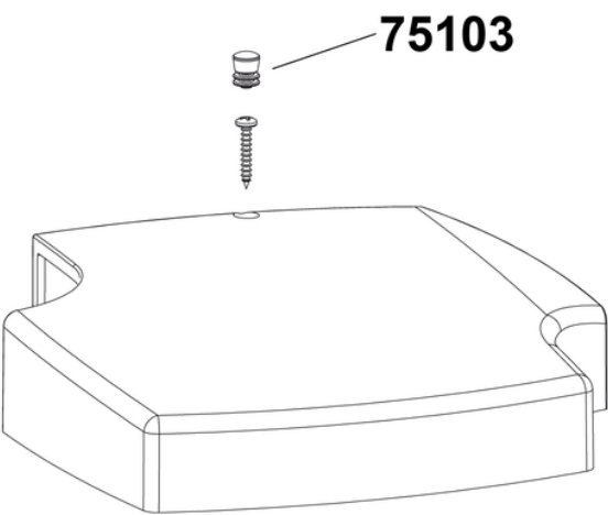
Tapa tornillos - CICLON L
