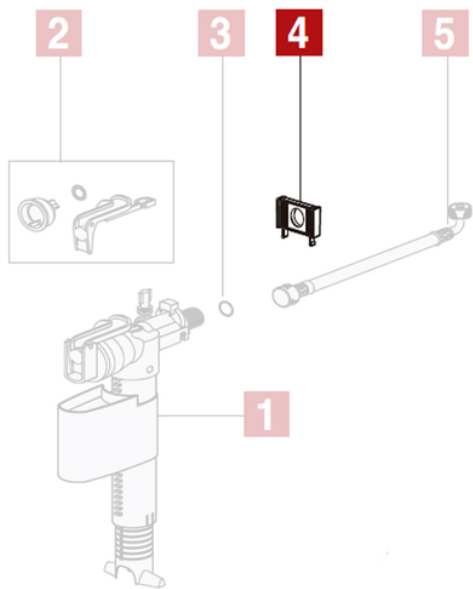
Soporte grifo flotador
