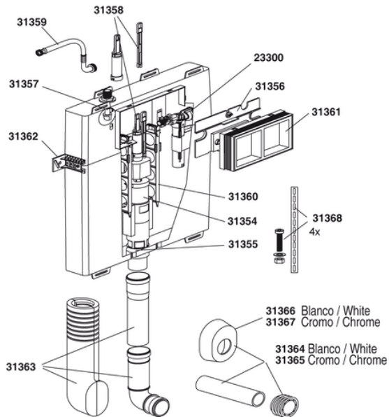
Latiguillo con juntas 3/8"
