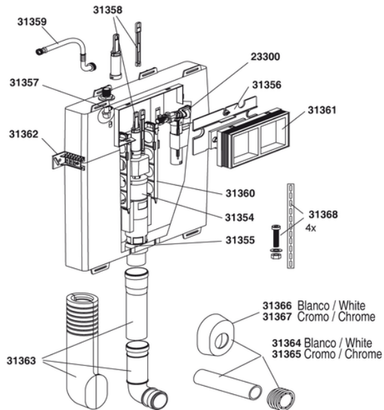
Mecanismo descarga S-800
